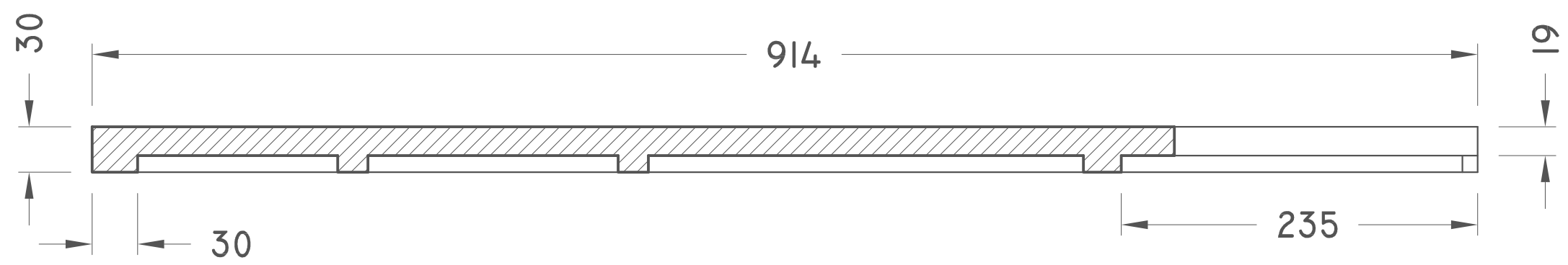
SECTION A-A
