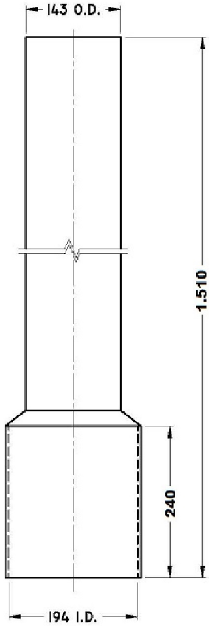
SECTION A-A
